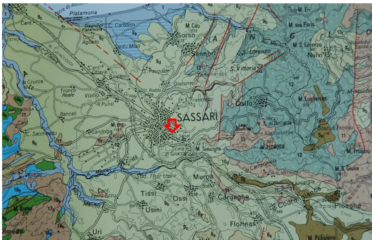
Figura 7 – Schema geologico del territorio circostante l'abitato di Sassari (stralcio della Carta Geologica della Sardegna – scala 1:200.000)
