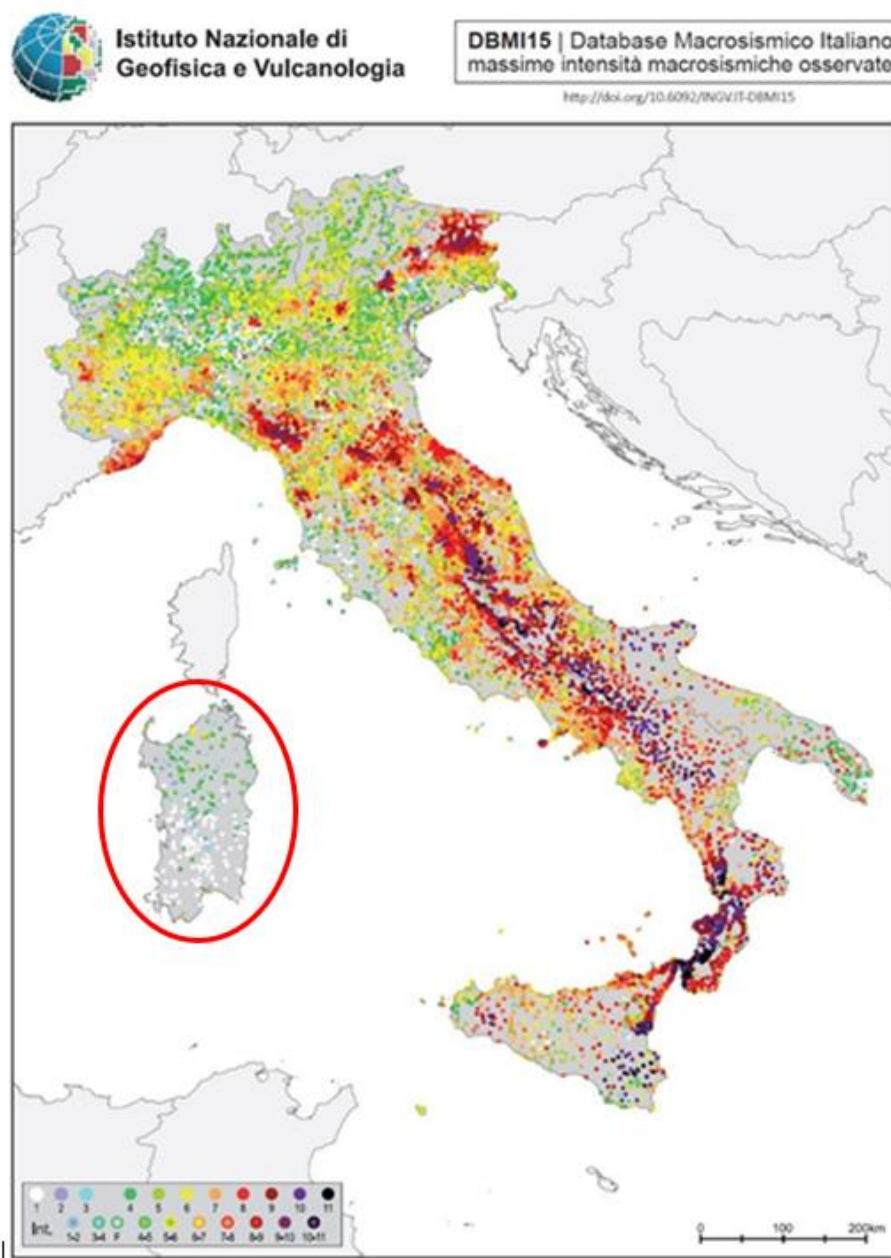
Figura 10 - Mappa con la localizzazione degli epicentri dei terremoti storici italiani riportati nel DBMI15 (fonte: INGV)
