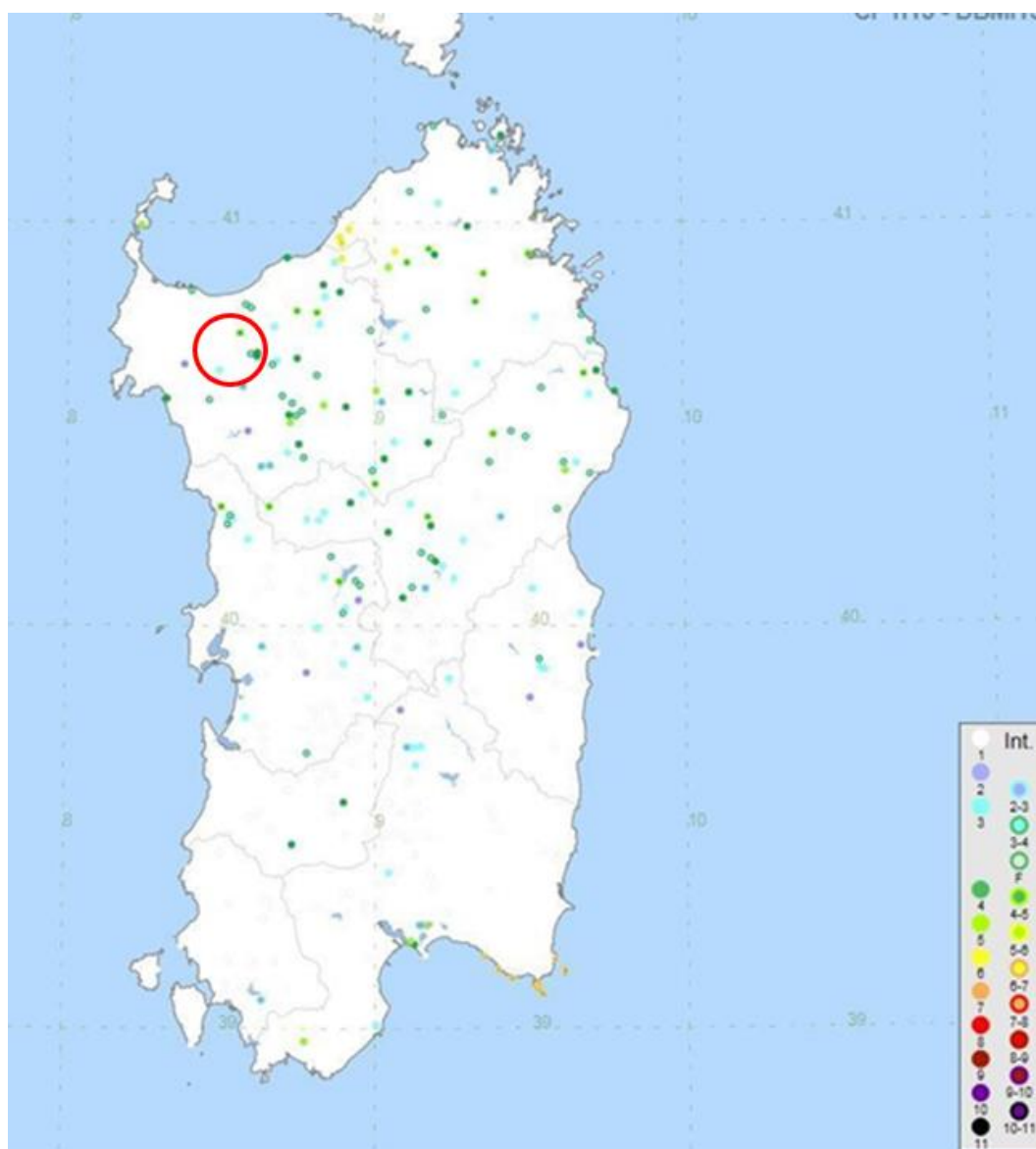
Figura 8 - Mappa con la localizzazione degli epicentri dei terremoti storici avvenuti in Sardegna (fonte: catalogo CPTI15, redatti da INGV)
