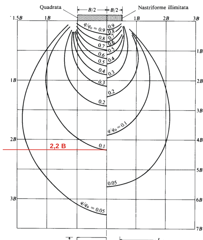
Figura 17 - Distribuzione delle tensioni nel sottosuolo per fondazione quadrata
