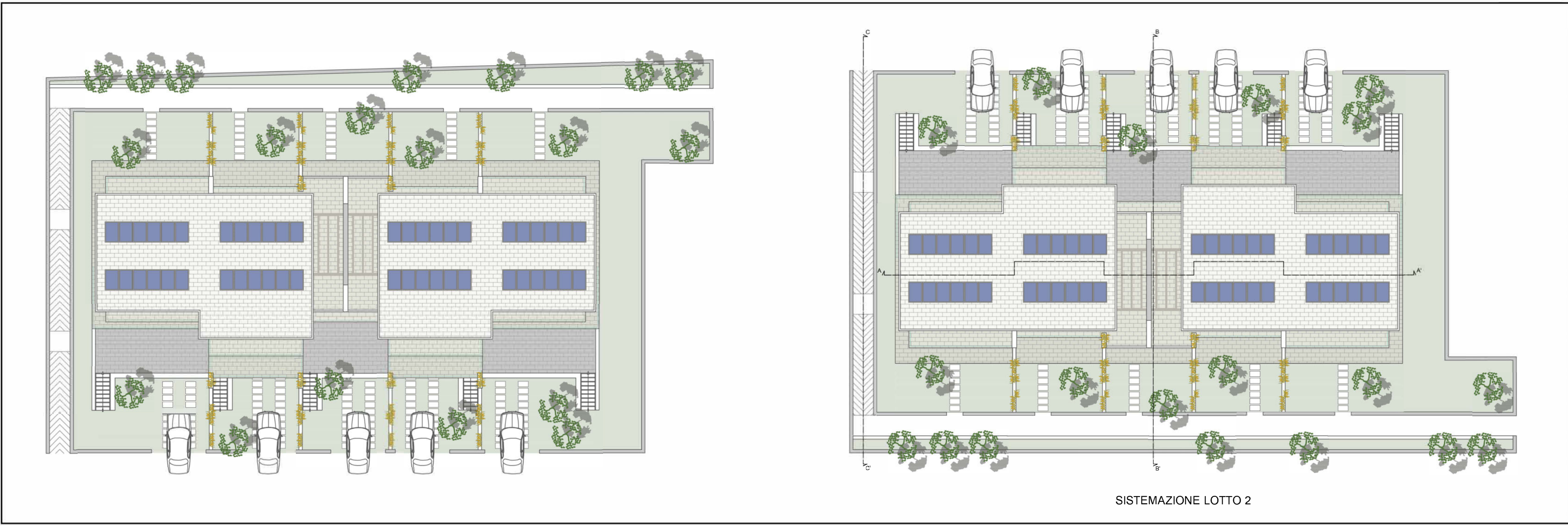
Piante e prospetti - Scala 1:200
