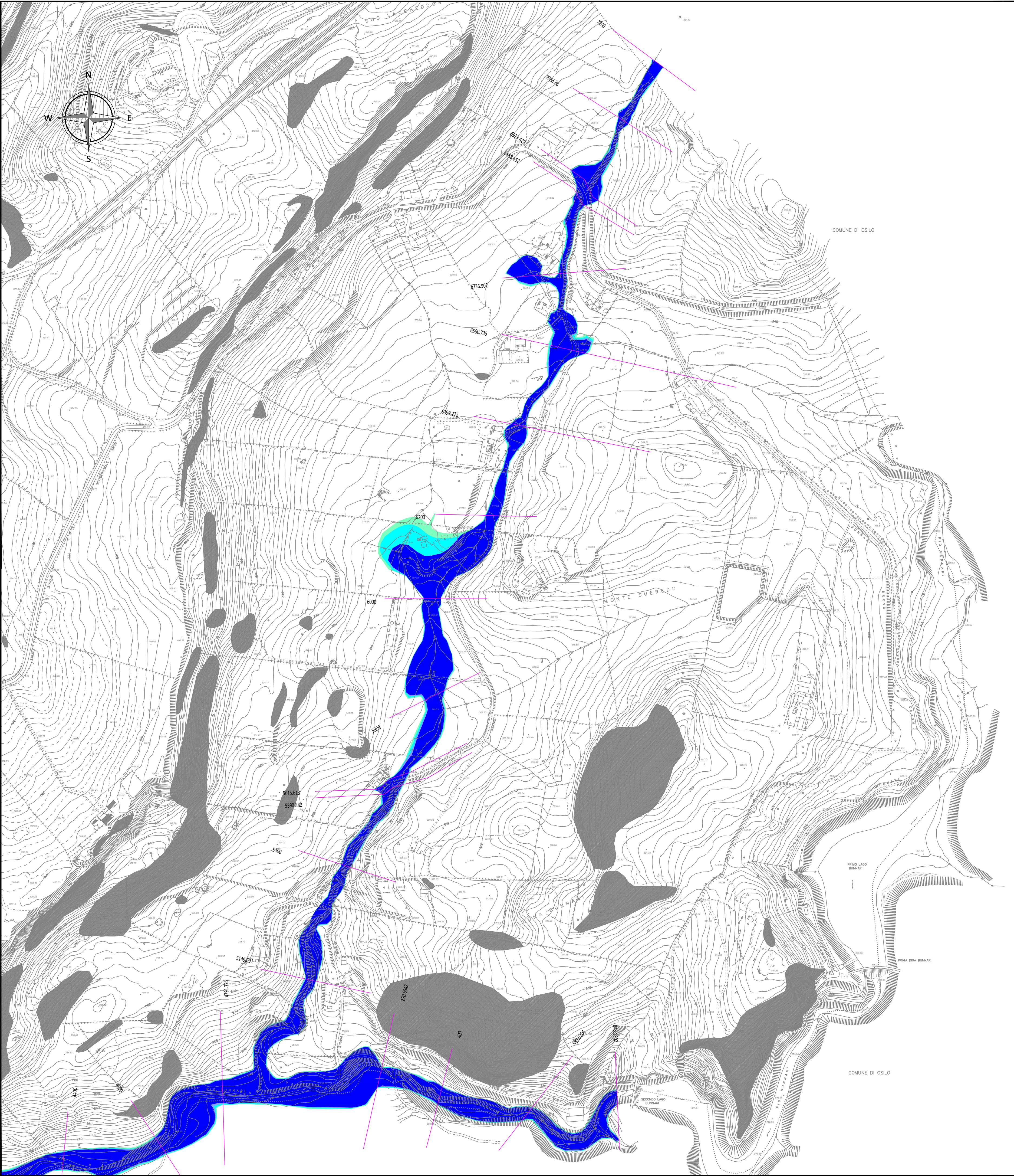
CARTA DELLA PERICOLOSITA' IDRAULICA - AREA EXTRAURBANA - SETTORE EST - RIO BUNNARI - SCALA 1:4.000
